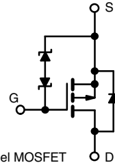
P-Channel MOSFET
